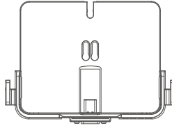
Βάση τοποθέτησης (×1)
